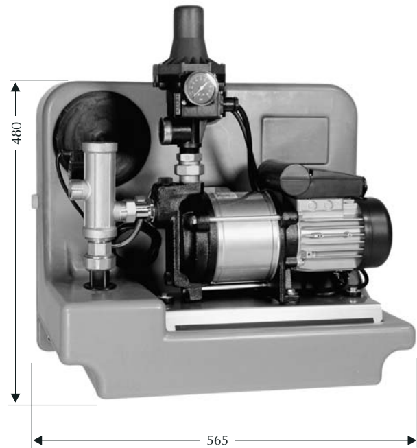
Bild 6 Maße und Anschlüsse
