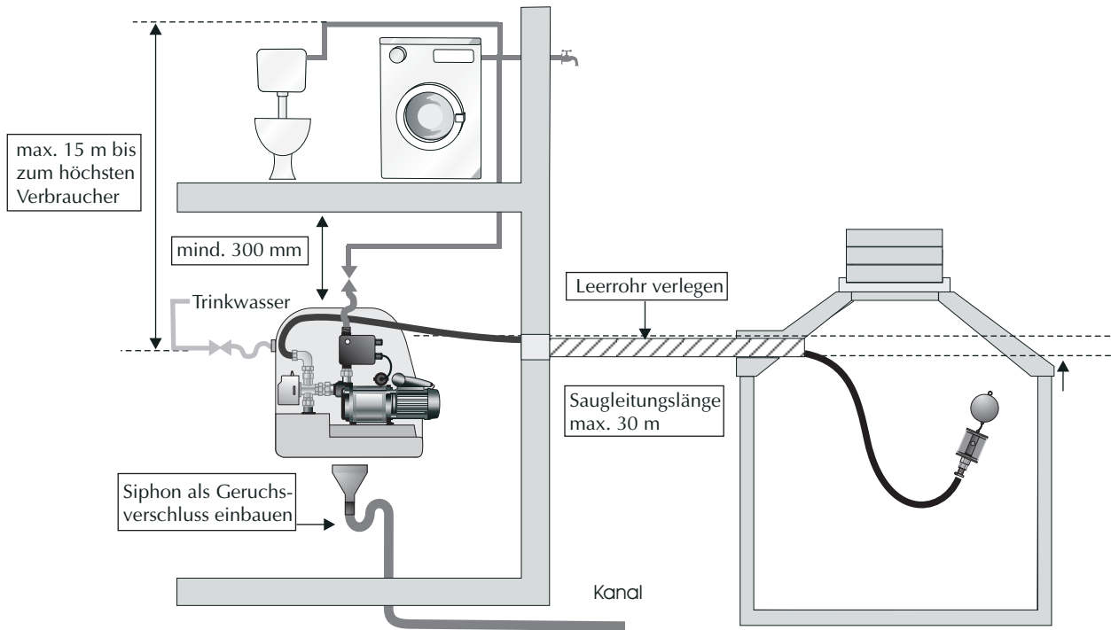
Bild 9 Hydraulischer Anschluss der Box V25K
